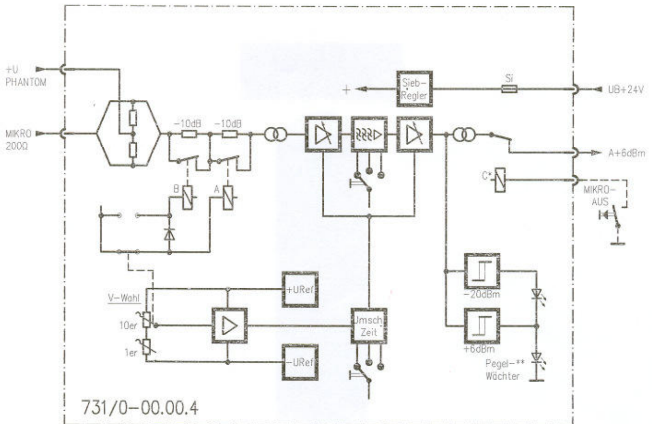
Blockschaltbild V976/0, V976/1, V976/5
