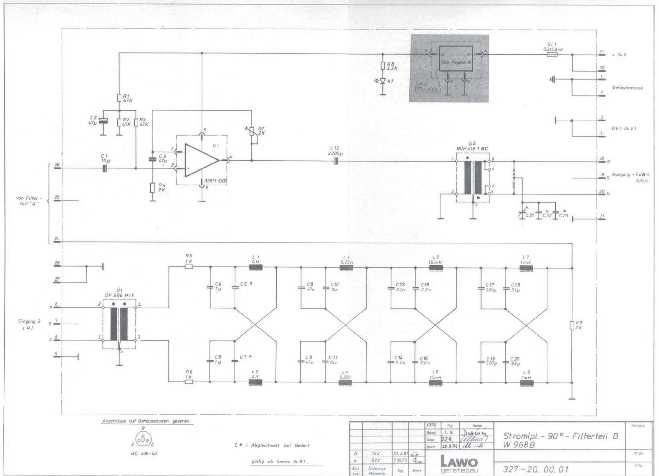
stromlaufplan c1-c2.tif
